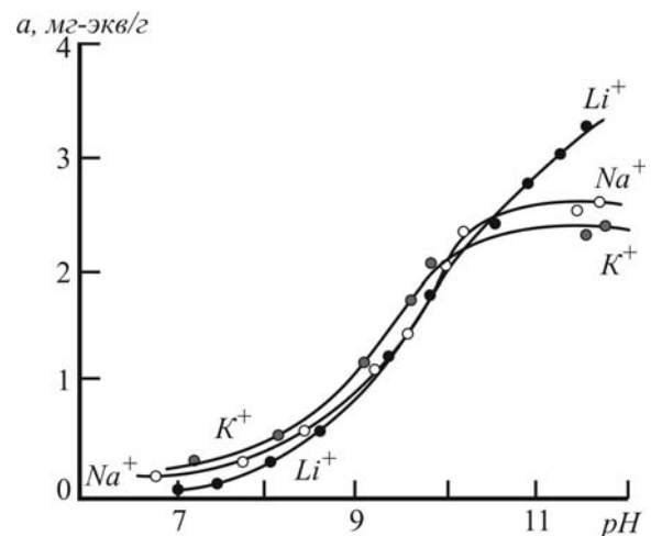
Рис. 7. Адсорбція катіонів лужних металів в області високих значень рН при титруванні силкагеля розчинами LiOH, NaOH, KOH [26]
