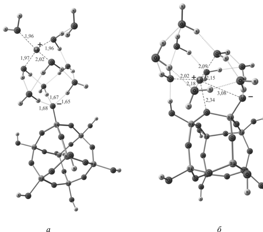
Рис. 8. Рівноважна структура комплексу, що містить молекулу \text{Si}_8\text{O}_{12}(\text{OH})_8 , дев'ять молекул води та катіон літію в стані з розділеними зарядами (а) та стані, що відповідає безпосередньому контакту катіона з депротонованою силанольною групою (б) [14]
