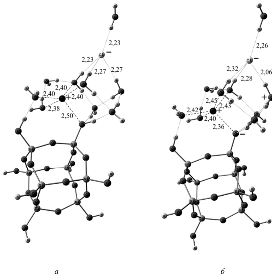
Рис. 4. Рівноважна просторова структура комплексу [\text{Si}_8\text{O}_{12}(\text{OH})_8, 9\text{H}_2\text{O}, \text{Na}^+, \text{Cl}^-] : а – стан з неіонізованою силанольною групою; б – стан з іонізованою силанольною групою [19]. Довжини зв'язків представлено в Å
