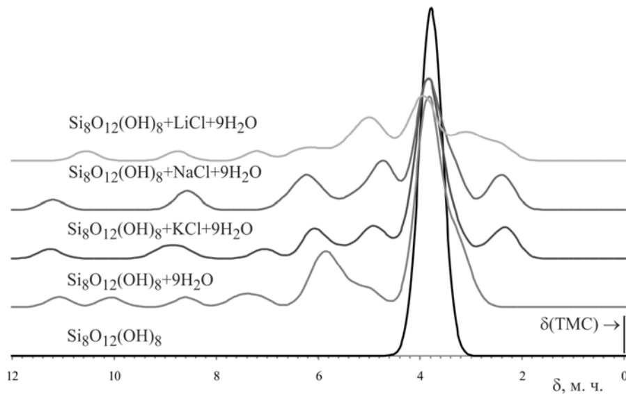
Рис. 6. Розраховані 1 H ЯМР-спектри комплексу [Si 8 O 12 (OH) 8 , 9H 2 O, K + , A - ] [25]
