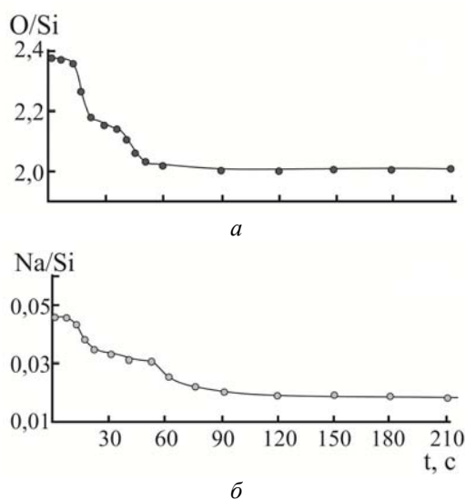
Рис. 3. Залежність атомних відношень O/Si (а) та Na/Si (б) від часу травлення іонами \text{Ag}^+ [18]
