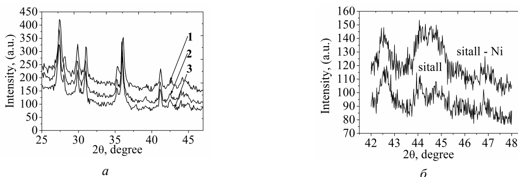
Рис. 1. Порівняння дифрактограм: а – ситалової підкладки (1), підкладки з осадженим Ni (2) та підкладки із шарами Ni та Gd 2 O 3 (3); б – ситалової підкладки, та підкладки з осадженим Ni в діапазоні 2θ = 42–48°
